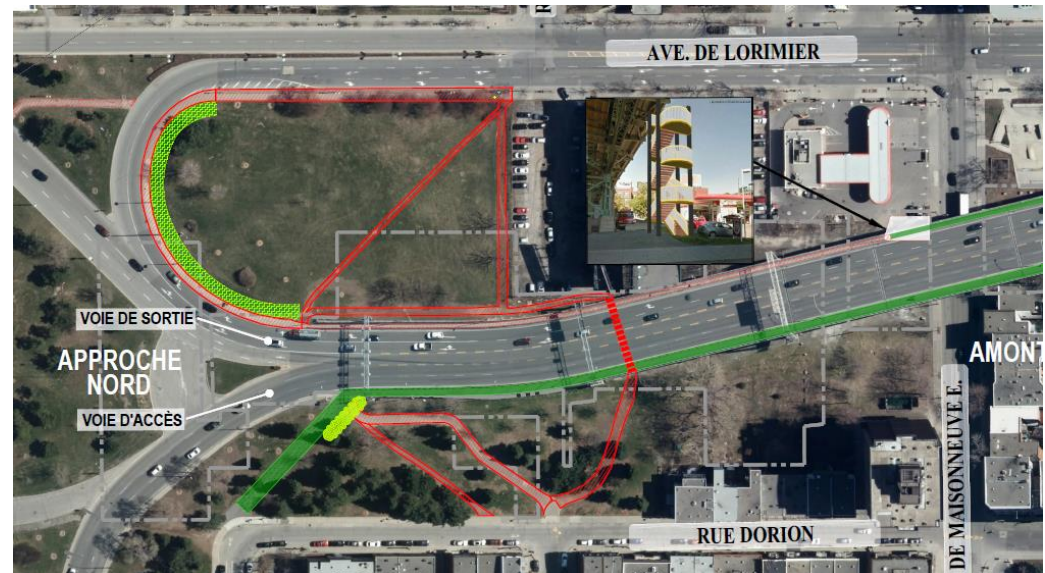
Esquisse préliminaire de l'escalier De Maisonneuve
