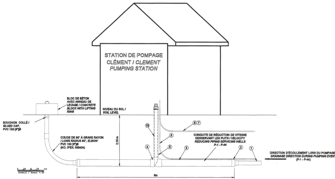
CONDUITE DE RALENTISSEMENT DE VITESSE - STATION DE POMPAGE CLÉMENT / VELOCITY REDUCING PIPE - CLEMENT PUMPING STATION ECHELLE / SCALE: 1:30
